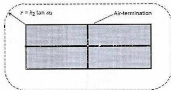
Hình B.4 - Vùng được bảo vệ bởi các dây dẫn dạng lưới tách biệt, xác định theo phương pháp góc bảo vệ và phương pháp quả cầu lăn
