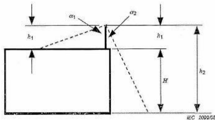
Hình B.1 - Vùng được bảo vệ bởi một điện cực thu sét thẳng đứng
