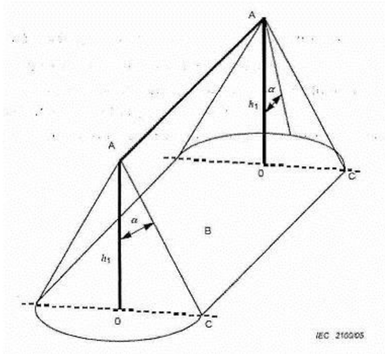
Hình B.3 - Vùng được bảo vệ bởi điện cực thu sét dạng dây
