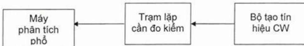
Hình D.5 - Sơ đồ đo xuyên điều chế đầu vào
