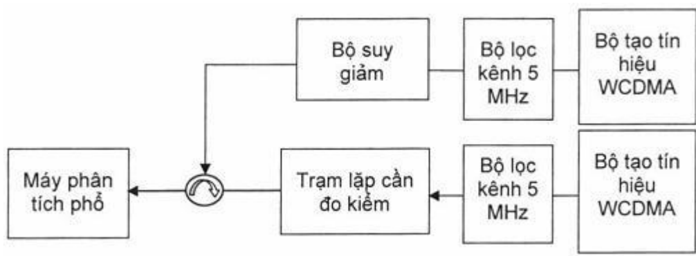
Hình D.6 - Sơ đồ đo xuyên điều chế đầu ra
