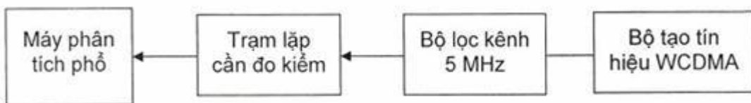
Hình D.4 - Sơ đồ đo phát xạ không mong muốn: phát xạ giả
