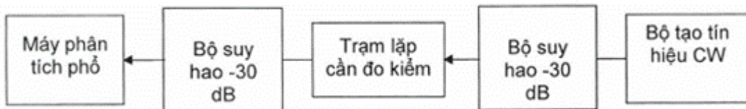
Hình D.2 - Sơ đồ đo tăng ích ngoài băng
