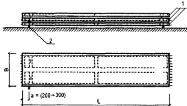
Hình 3 - Kê xếp tấm sàn bê tông cốt thép ứng lực trước
