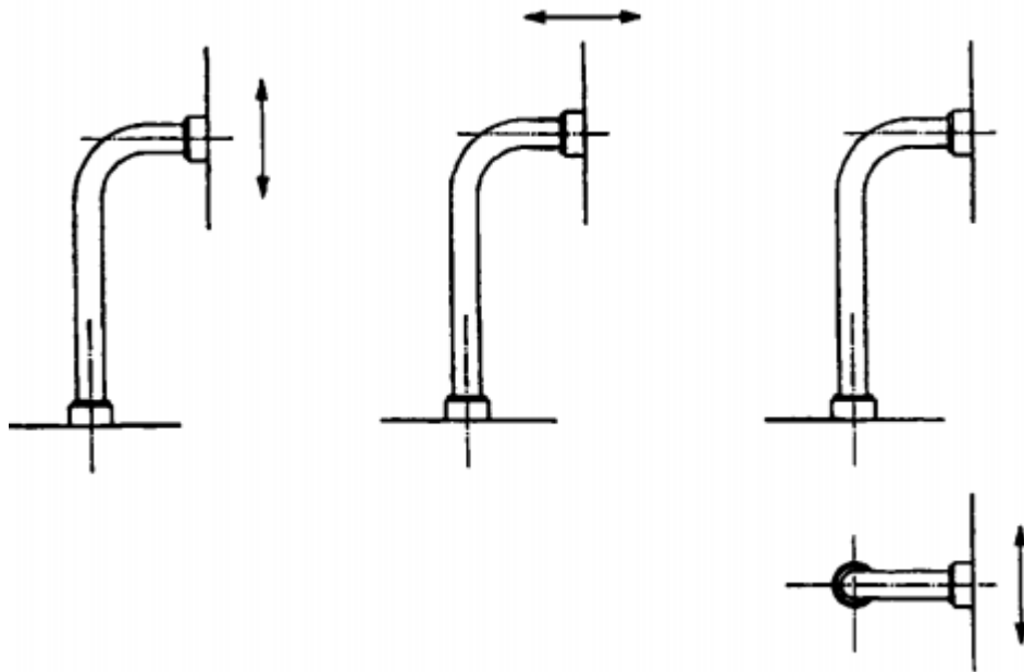
Hình C.1 - Các hướng rung của mẫu thử
