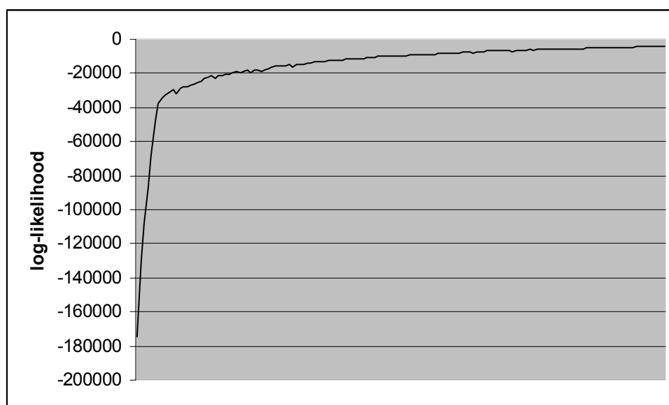
Hình 8: Quá trình tăng likelihood qua 150 bước lặp
