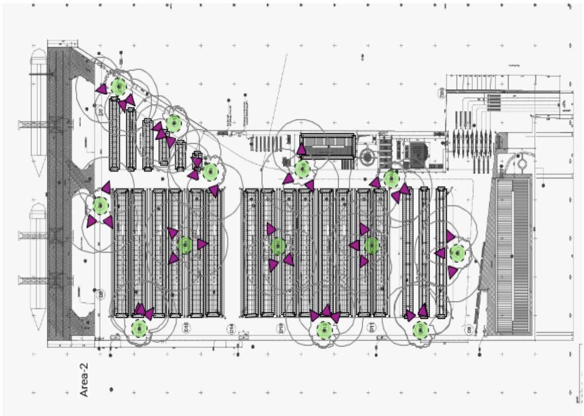
Hình 3-14: Sơ đồ bố trí lắp đặt thiết bị
