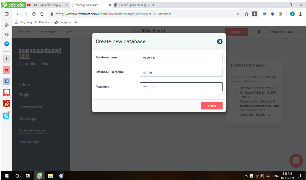
Hình 2.11 Tạo database
