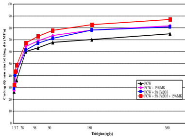
Hình 4.13: Ảnh hưởng của oxyt màu sắt Fe 2 O 3 đến sự phát triển R n BTTT mác 60MPa theo τ
