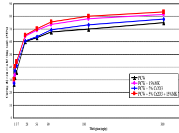
Hình 4.9: Ảnh hưởng của oxyt crôm Cr 2 O 3 đến sự phát triển R n BTTT mác 60MPa theo τ
