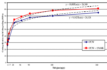
Hình 4.4: Ảnh hưởng của 15% MK đến sự phát triển cường độ nén của BT trắng mác 60MPa
