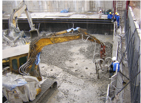
Hình 4. Đảm bê tông bằng đầm rung chuyên dụng tại đập CVC Sesan 3
