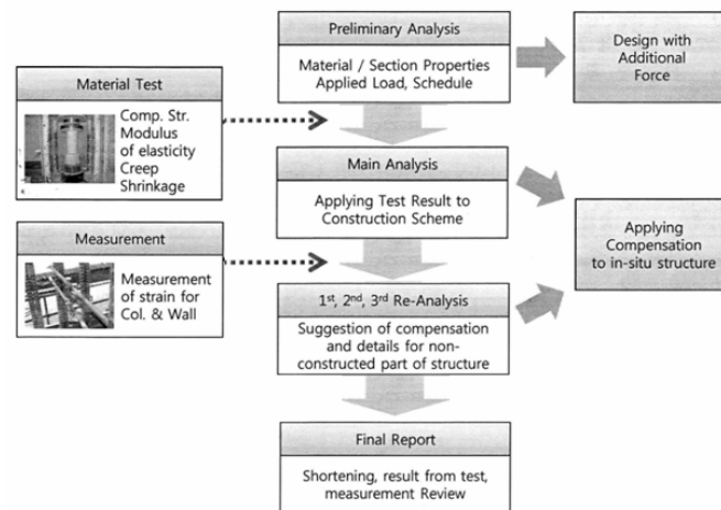
Hình 4. Keangnam - Quy trình thiết kế có kể đến hiệu ứng co ngắn cột [6]
