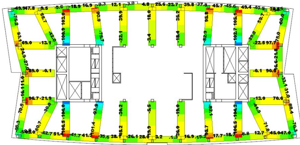
Hình 3. Hotel tower – Giá trị mô men phát sinh tại các dải sàn tầng 70 do độ vênh co ngấn gây ra, kNm/m [7]
