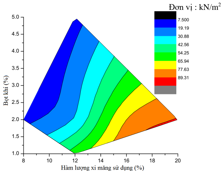
Hình 3. Cường độ kháng nén không nở hông của đất nhẹ gia cố theo hàm lượng xi măng và thể tích bột khí
